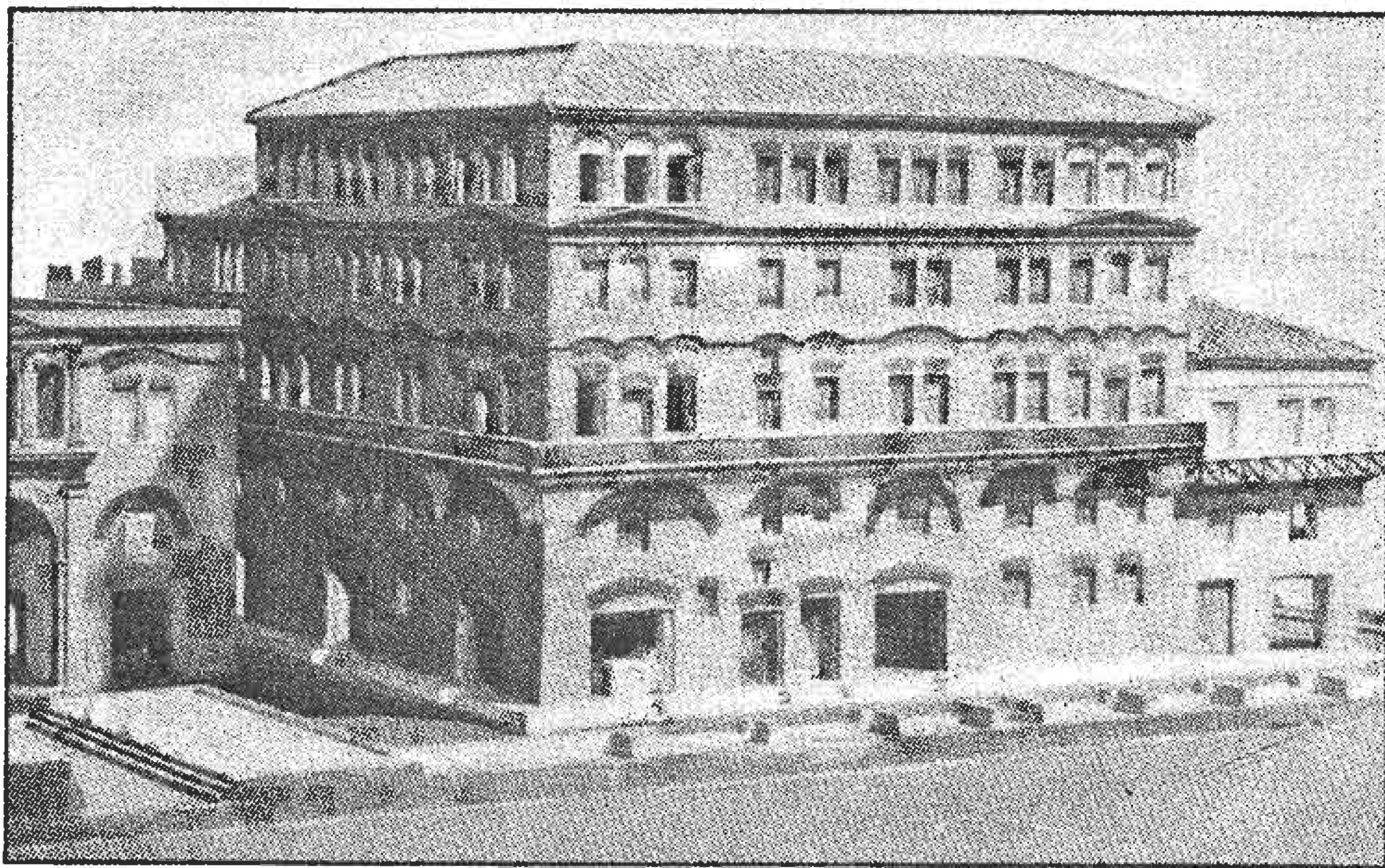
Инсула (реконструкција)
