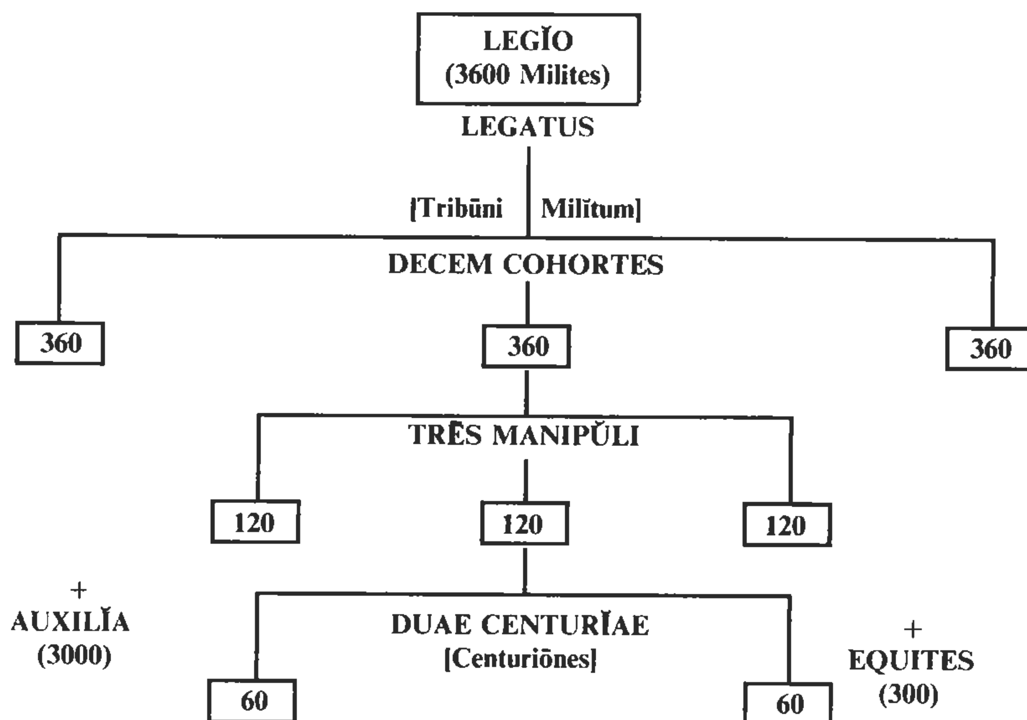
Устројство легије
